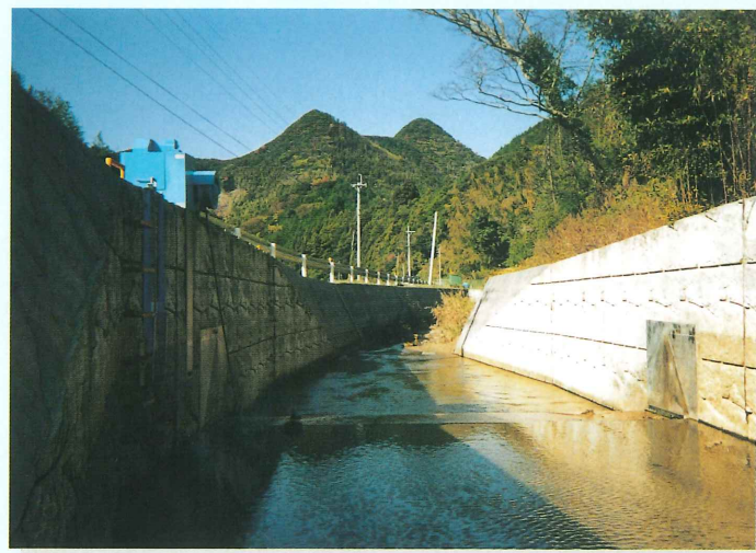
（ユニット式転倒ゲート）
