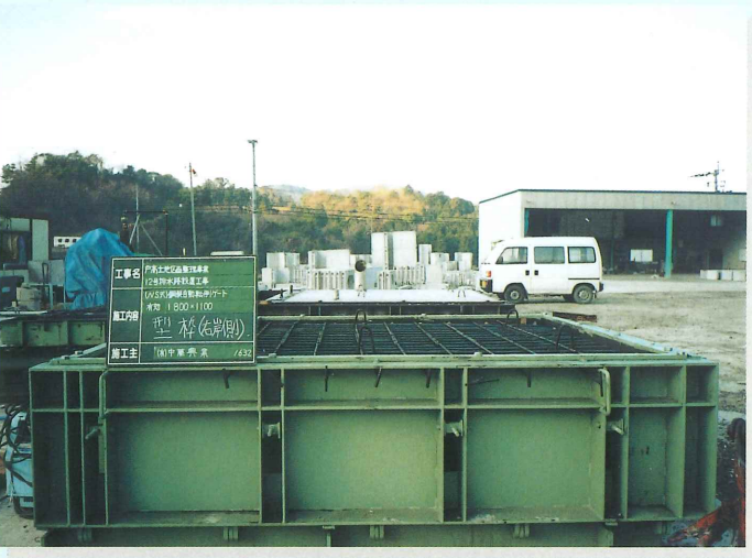
（型枠組付）
