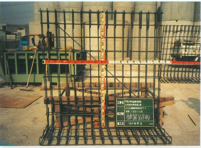
（鉄筋配筋）
