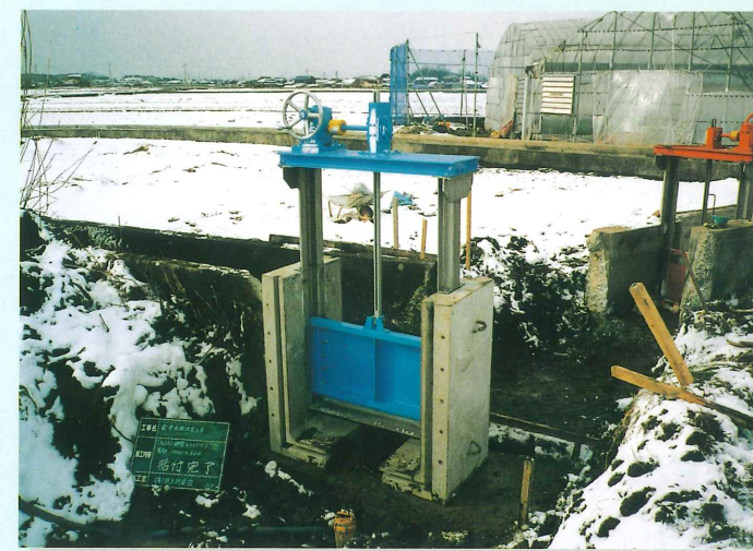
(現場施工完成)
