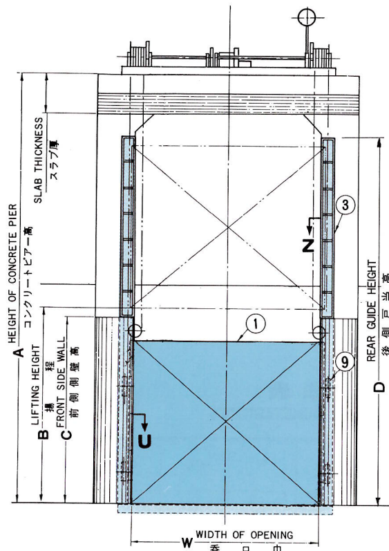
FRONT VIEW 正面図
