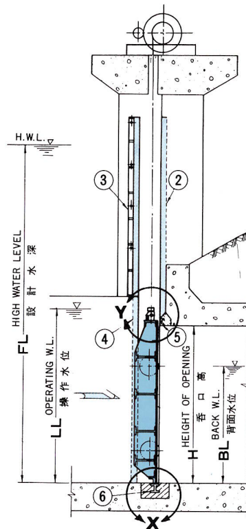
SECTION 断面図
